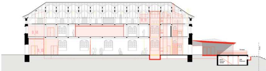
LÄNGSSCHNITT L-L 1:200
