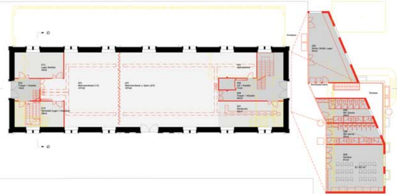
ERDGESCHOSS - Wechselveranstaltungen 1:200
